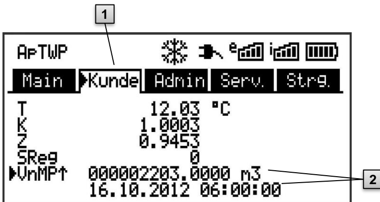
Abb. 28: Register „Kunde“
