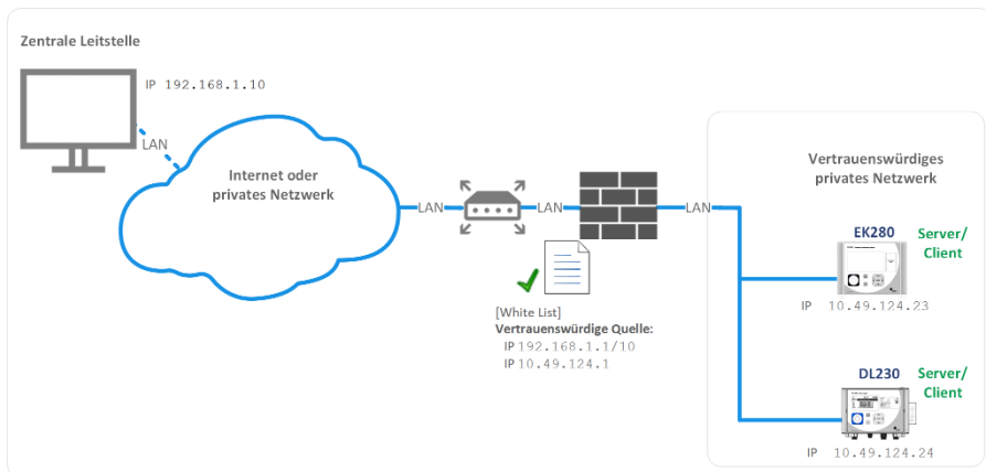
Abb. 1: Router und Firewall zwischen Messanlage und Leitstelle – Beispiel
